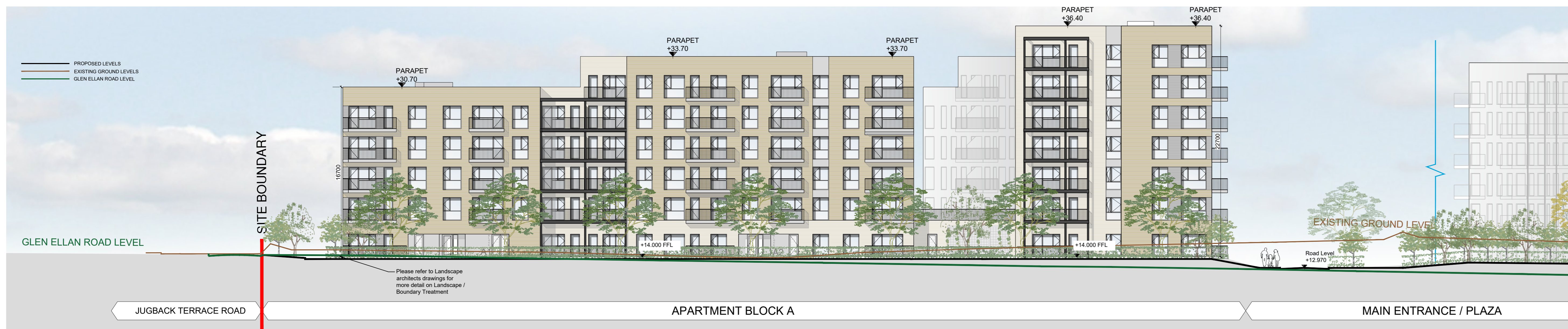
SECTION A-A
